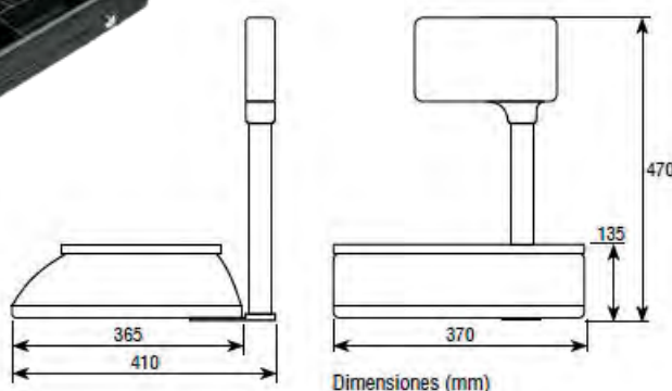
Dimensiones (mm)
