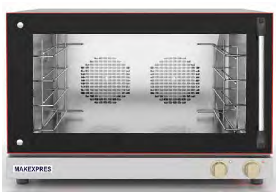
4 BANDEJAS DE 600 x 400 mm. - 0-4-GN-1/1-GASTRONOMÍA CPL-64 APERTURA LATERAL PUERTA BANDERA
